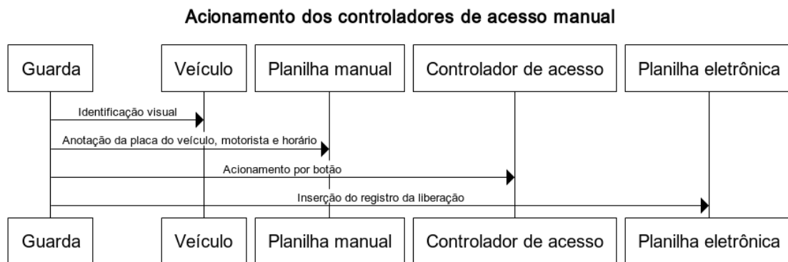
Figura 14 - Diagrama de acionamento dos controladores de acesso manual
