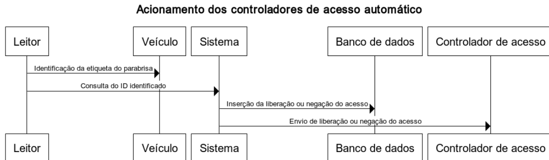
Figura 15 - Diagrama de acionamento dos controladores de acesso automático
