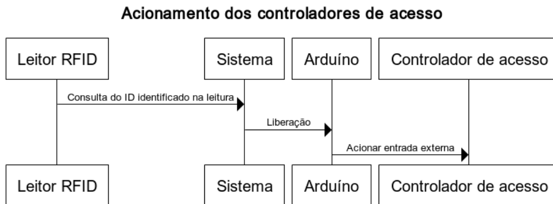
Figura 10 - Diagrama de acionamento dos controladores de acesso
